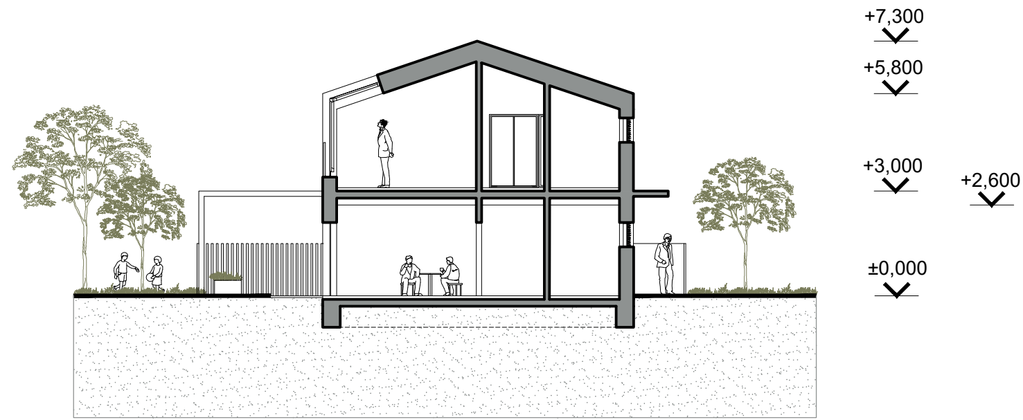
PRIEČNY REZ
