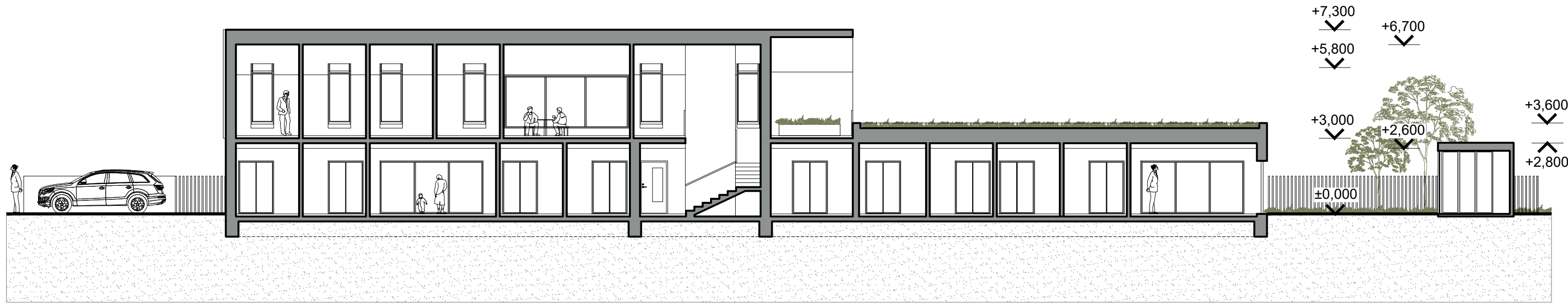
POZDĹŽNY REZ
